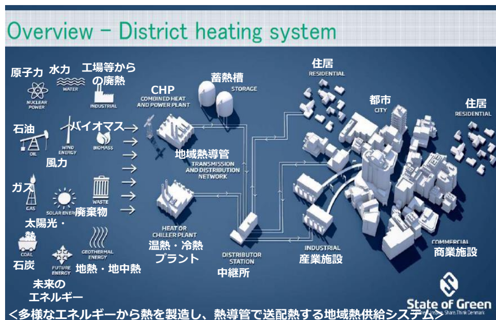
地域熱供給の全体概念図
