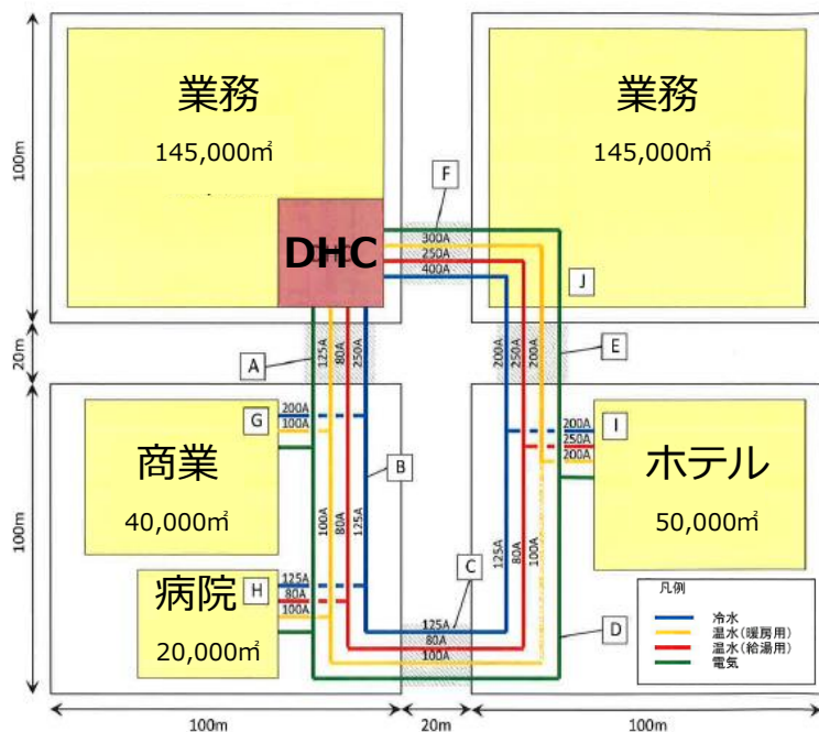
モデル概念図 熱電一体供給モデル
